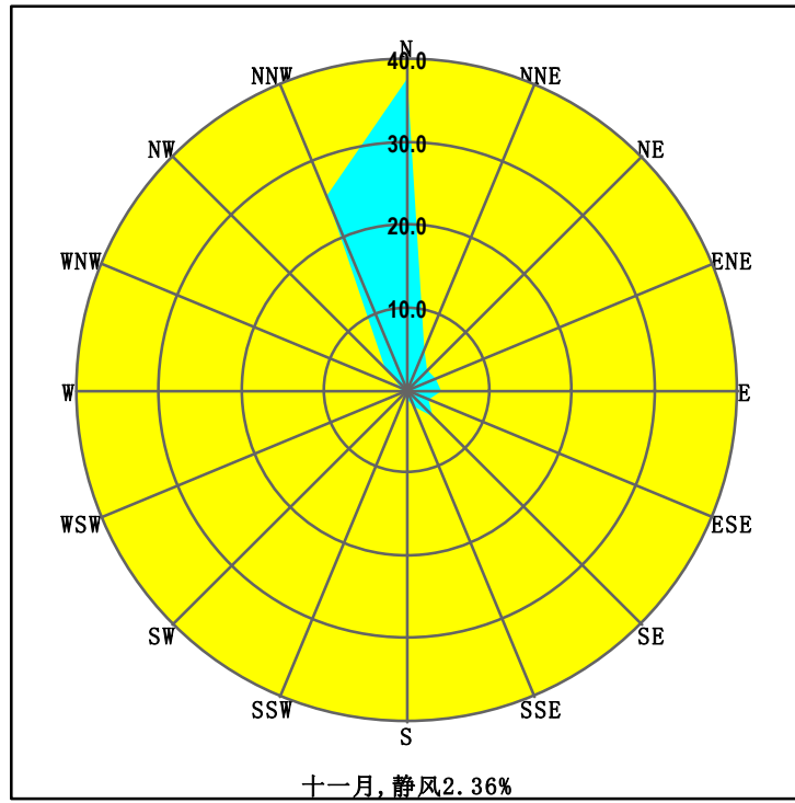
图3 广州（黄埔）国家基本气象站 2022 年 11 月 16 方位逐时风频玫瑰图
