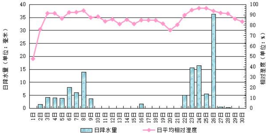
图 2 广州（黄埔）国家基本气象站 2022 年 11 月份逐日相对湿度和降水量
